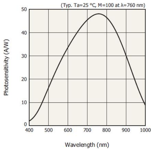
APD410A 响应曲线
