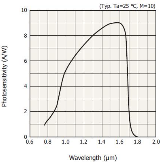
APD410C 响应曲线
