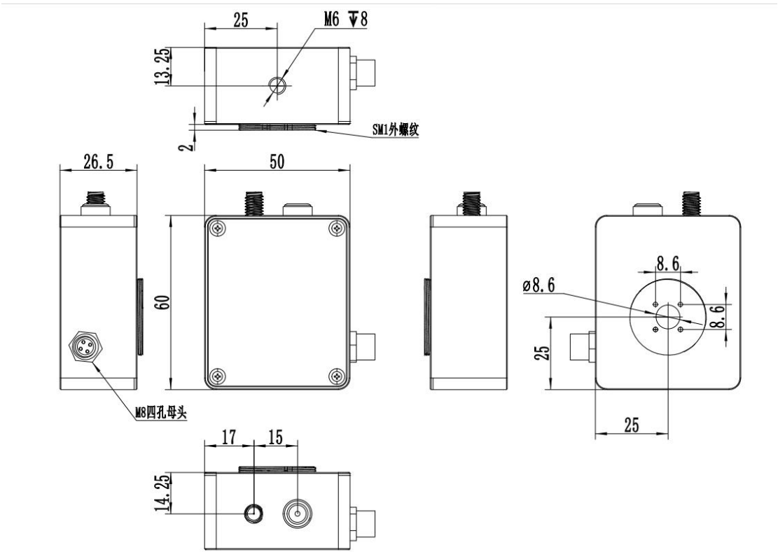
SM1 外螺纹数字可调增益结构（选配）
