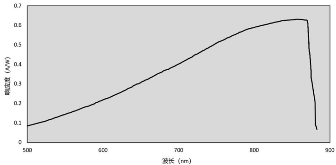
HS61A 响应曲线
