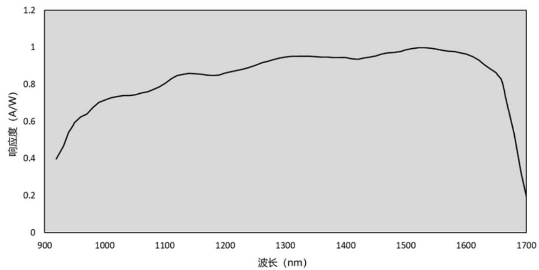
HS61C 响应曲线
